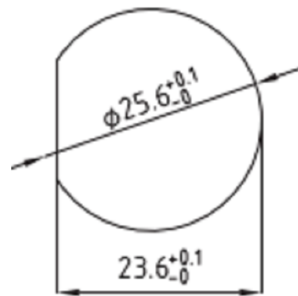
面板开孔尺寸
